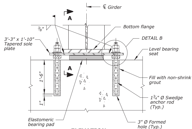
ELEVATION Scale: 1" = 1'-0"
